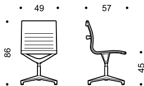
UNA 105. Swivel chair without arms return mechanism 4-star base on glides Sedia girevole senza braccioli meccanismo di ritorno base a 4 razze con finalini
