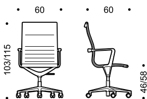
UNA 118. Swivel chair high back with arms height adjustable 5-star base on castors Sedia girevole schienale alto con braccioli regolabile in altezza base a 5 razze con ruote
