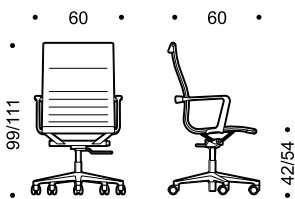
UNA 119. Swivel chair high back with arms height adjustable tilting mechanism 5-star base on castors Sedia girevole schienale alto con braccioli regolabile in altezza meccanismo di oscillazione base a 5 razze con ruote
