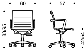
UNA 117. Swivel chair with arms height adjustable tilting mechanism 5-star base on castors Sedia girevole con braccioli regolabile in altezza meccanismo di oscillazione base a 5 razze con ruote
