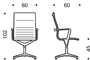
UNA 115. Swivel chair high back with arms return mechanism 4-star base on glides Sedia girevole schienale alto con braccioli meccanismo di ritorno base a 4 razze con finalini
