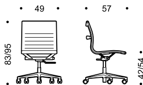
UNA 116. Swivel chair without arms height adjustable tilting mechanism 5-star base on castors Sedia girevole senza braccioli regolabile in altezza meccanismo di oscillazione base a 5 razze con ruote
