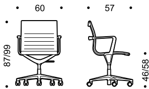
UNA 109. Swivel chair with arms height adjustable 5-star base on castors Sedia girevole con braccioli regolabile in altezza base a 5 razze con ruote
