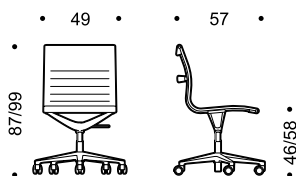
UNA 106. Swivel chair without arms height adjustable 5-star base on castors Sedia girevole senza braccioli regolabile in altezza base a 5 razze con ruote
